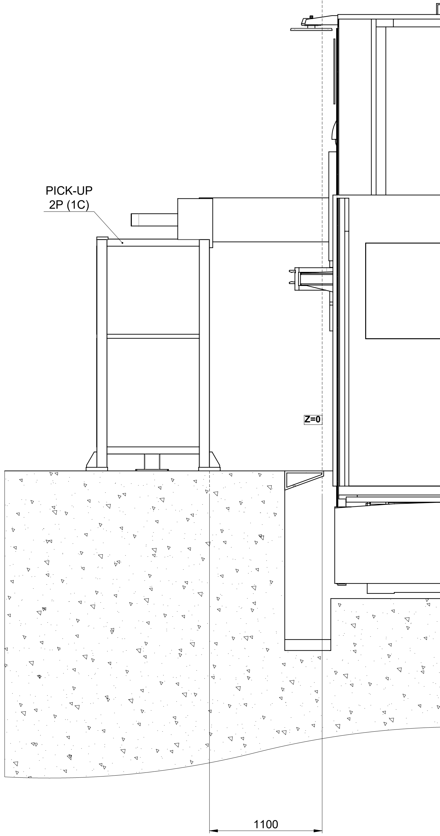
A-A 270°
